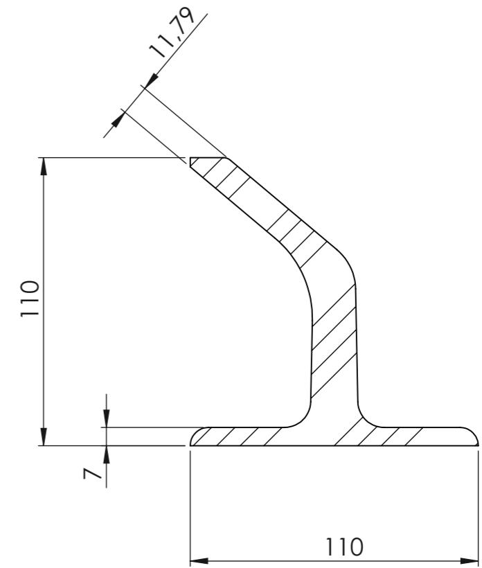
SEZIONE A-A
